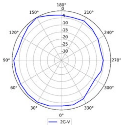
2.4 GHz (Vertical)
