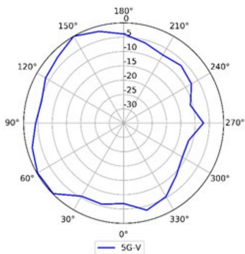
5 GHz (Vertical)
